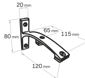
Nosník Elegance dvojitý 12 cm
