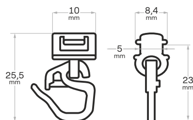
Nacvakávací jezdec s háčkem
