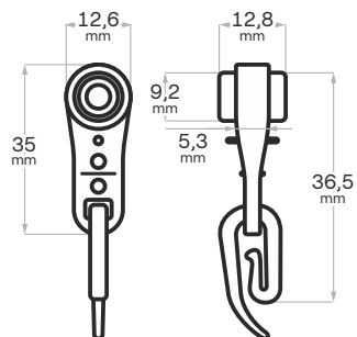
Ložiskový jezdec s háčkem
