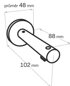
Nosník Deco jednoduchý 10 cm
