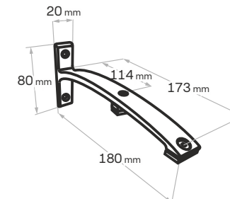
Nosník Elegance dvojitý prodloužený 18 cm
