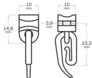
Jezdec + šnekový háček
