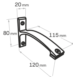
Nosník Elegance jednoduchý 12 cm
