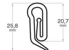
Šnekový háček malý
