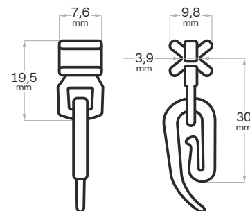
Jezdec TFL + šnekový háček
