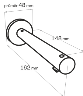
Nosník Deco jednoduchý prodloužený 16 cm
