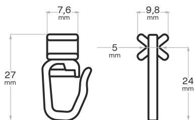
Jezdec s háčkem
