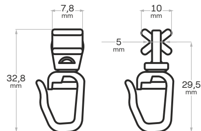
Otočný jezdec s háčkem
