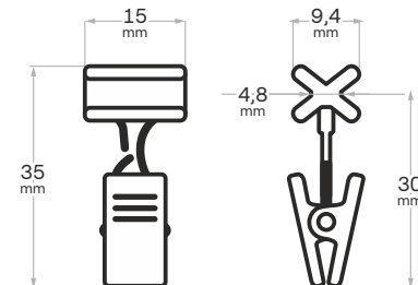
Jezdec s žabkou
