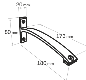
Nosník Elegance jednoduchý prodloužený 18 cm
