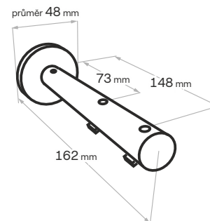
Nosník Deco dvojitý 16 cm
