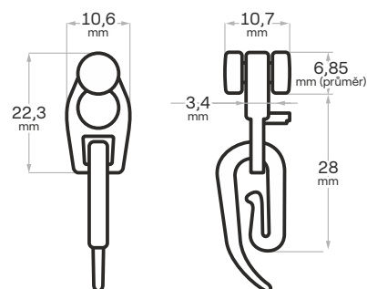
Kolečkový jezdec + šnekový háček
